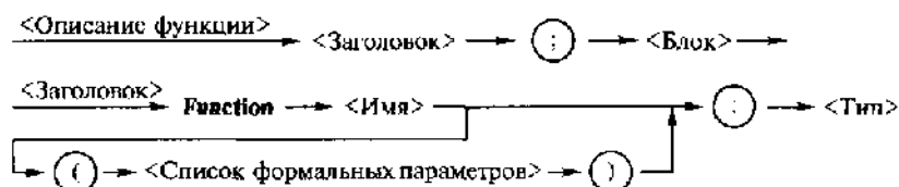
Рис. 2.23. Синтаксическая диаграмма описания функции
