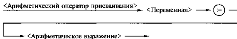
Рис. 2.10. Структура арифметического оператора присваивания
