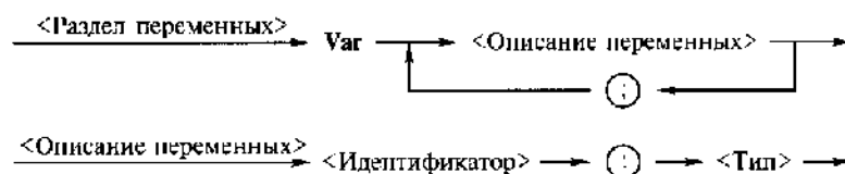
Рис. 2.3. Структура раздела переменных
