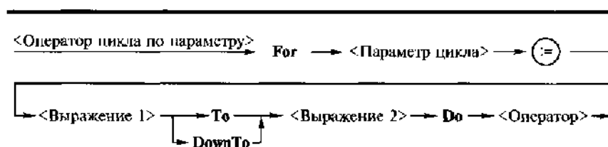
Рис. 2.20. Синтаксическая диаграмма цикла с параметром
