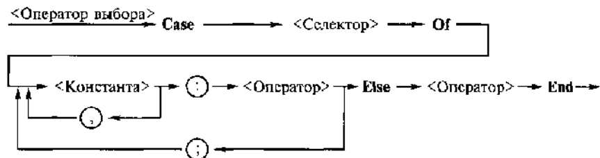
Рис. 2.15. Синтаксическая диаграмма оператора выбора
