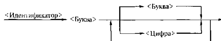
Рис. 2.1. Синтаксическая диаграмма идентификатора
